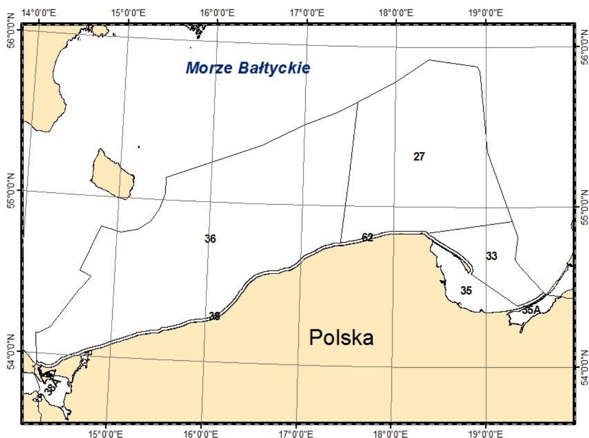
Rys. 3. Podakweny Morza Bałtyckiego wyznaczone w ramach HELCOM CORESET BD 2/2011 (źródło: PMS)
