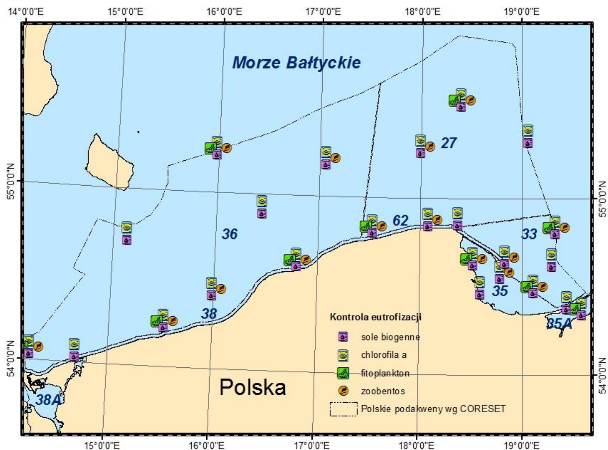
Rys. 8 Lokalizacja stanowisk badań fitoplanktonu, makrozoobentosu oraz soli biogenicznych w ramach cechy 5 na polskich obszarach morskich. (źródło: PMŚ)
