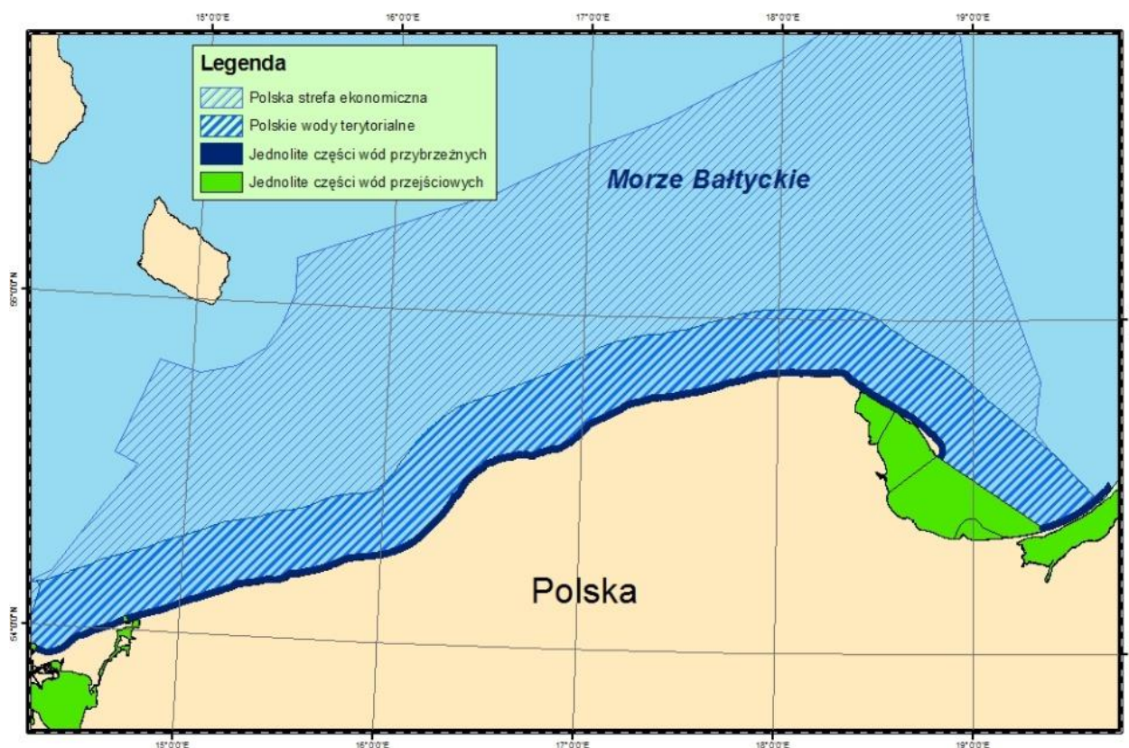
Rys. 2. Polskie obszary morskie poddane ocenie wstępnej zgodnie z art. 8 Ramowej Dyrektywy ws. Strategii Morskiej (źródło: PMŚ)
