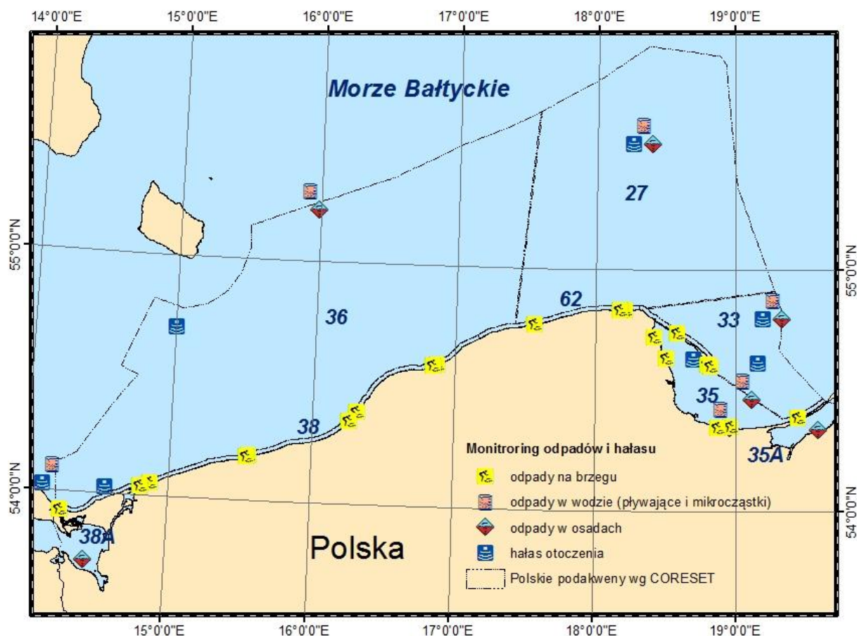
Rys. 12. Lokalizacja stanowisk badań odpadów i hałasu podwodnego na polskich obszarach morskich. (źródło: PMŚ)
