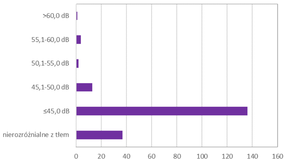
Wykres VI.2. Ilość pomiarów wykonanych w 2020 r. z wynikiem oznaczonym w poszczególnych zakresach – pora – pora nocna
