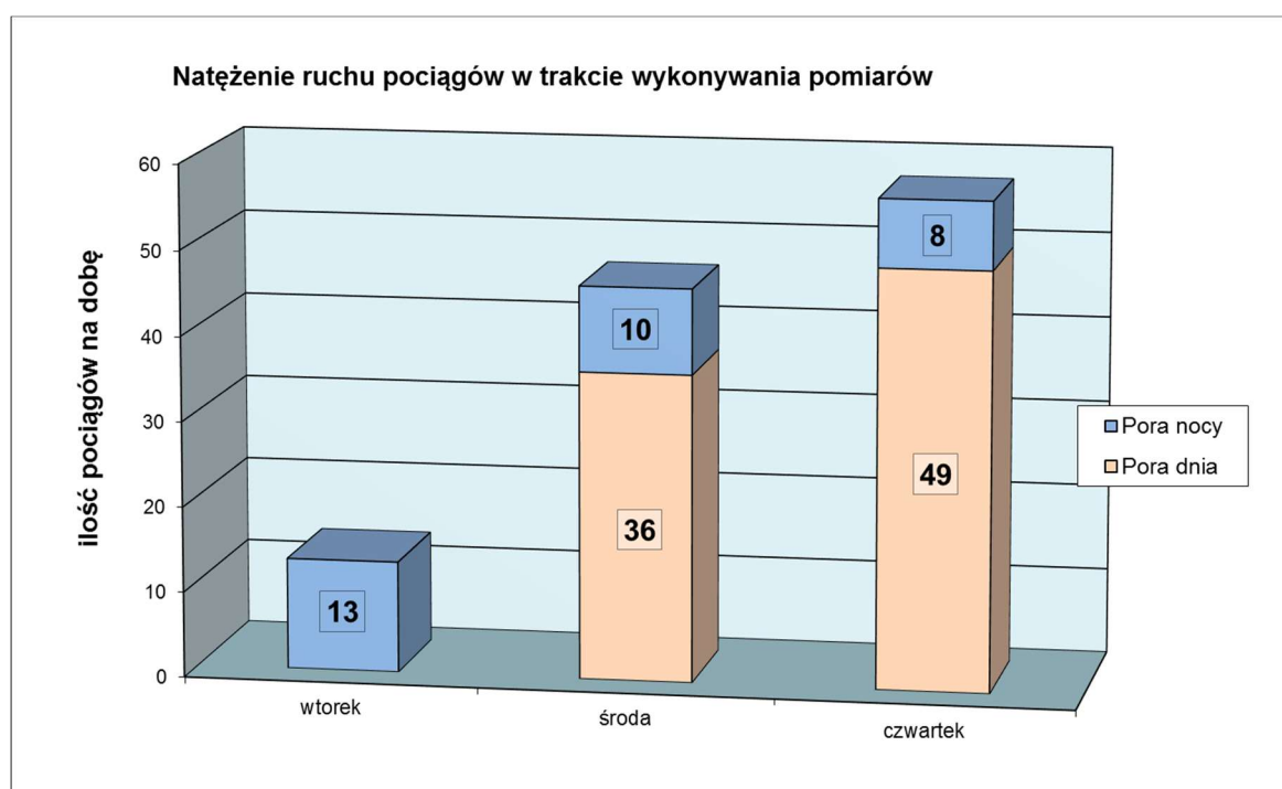
Ryc. 5. Natężenie ruchu pociągów w czasie trwania sesji pomiarowej na badanym odcinku linii kolejowej nr 140, Nędza, ul. Leśna.
