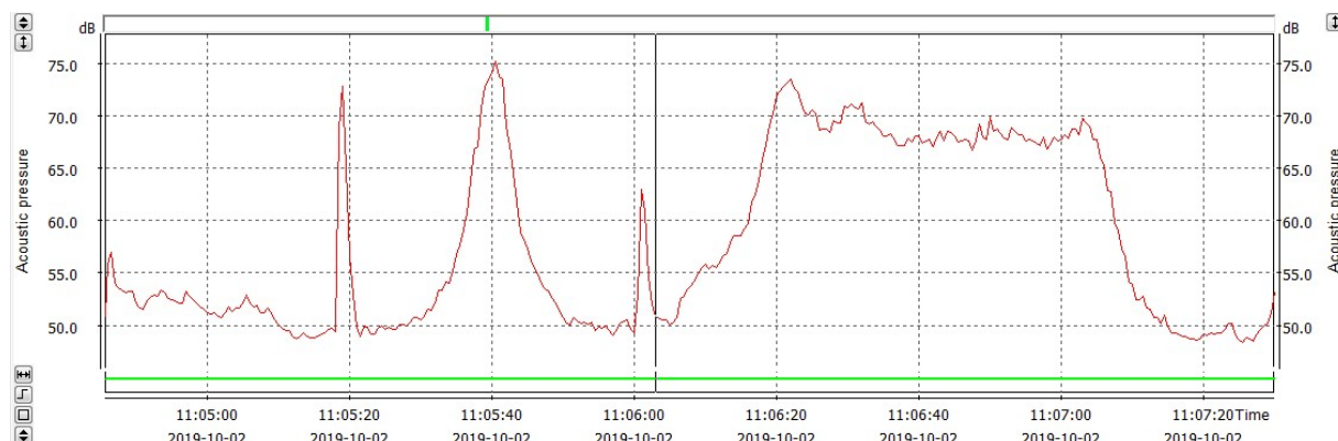
Ryc. 4. Przebieg zmian poziomu dźwięku A w funkcji czasu t dla przejazdu pociągu osobowego (11:05) oraz towarowego (11:06), zarejestrowane w punkcie obserwacji dźwięku PR1, Nędza, rejon ul. Leśnej.
