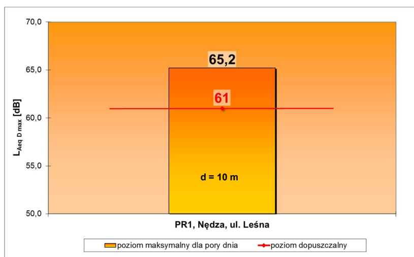
Ryc. 2. Wartość wskaźnika L_{Aeq D}^{2dmax} dla rozpatrywanego punktu referencyjnego oraz jego porównanie z obowiązującą wartością poziomu dopuszczalnego, Nędza, 2019 rok.
