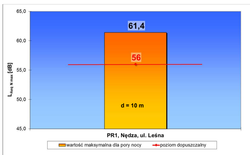
Ryc. 3. Wartość wskaźnika L_{Aeq N}^{3dmax} dla rozpatrywanego punktu referencyjnego oraz jego porównanie z obowiązującą wartością poziomu dopuszczalnego, Nędza, 2019 rok.
